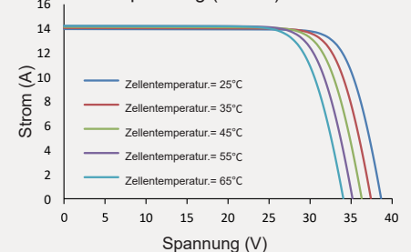
Strom/Spannung (430 W)
